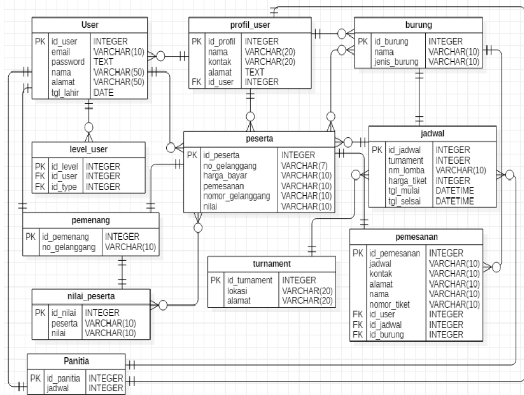
Gambar 5. ER Diagram
